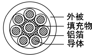
编码器电缆线断面
