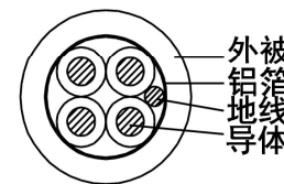
电机电缆线断面
