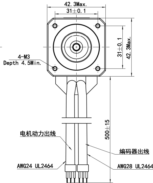
编码器 Encoder detail 型号 (Model): AM4096-1024P/R 分辨率: 1024线
